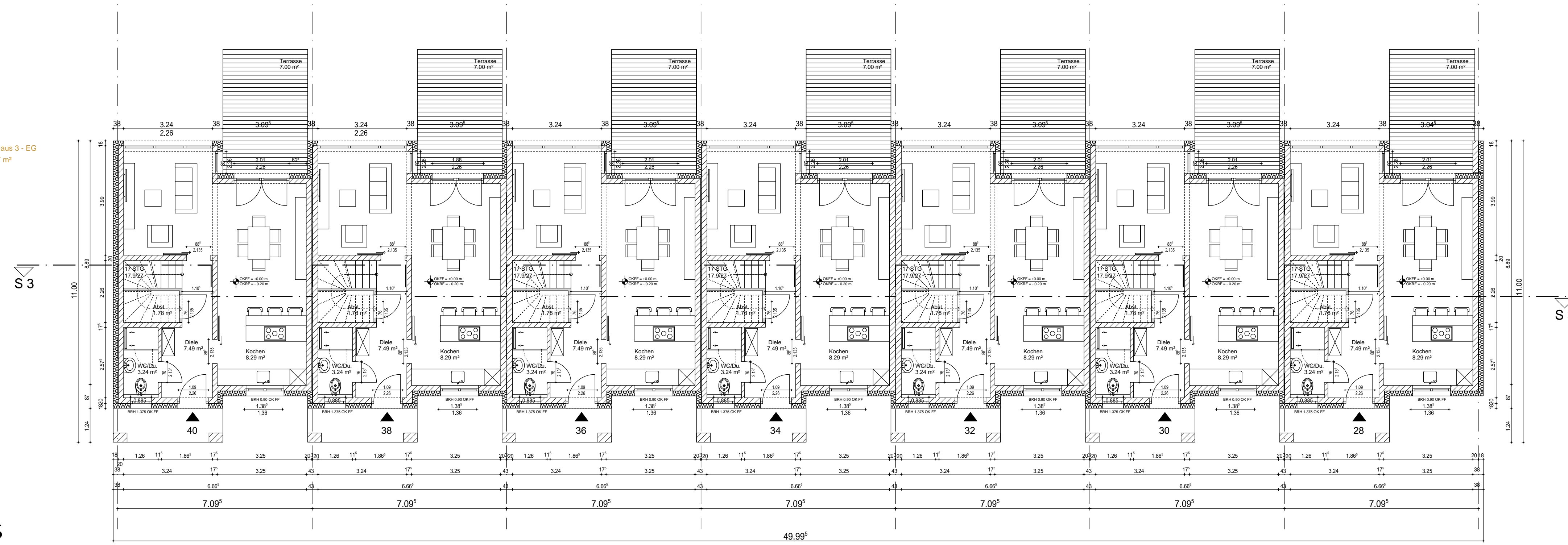
ERDGESCHOSS
