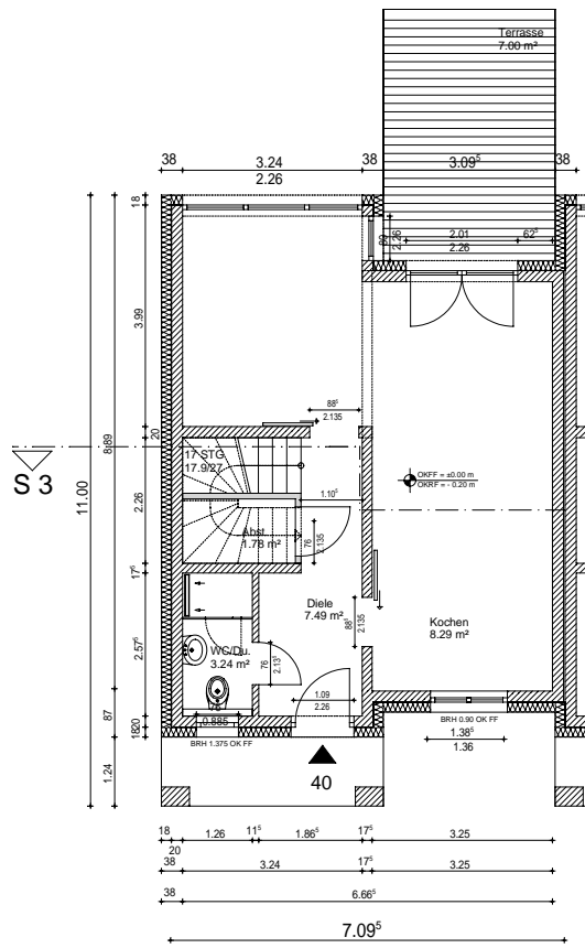
Haus 3 RH 20 - Erdgeschoss
