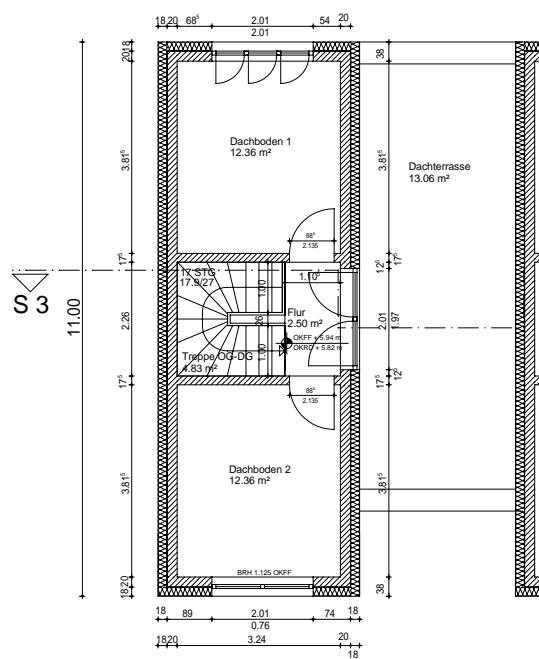
Haus 3 RH 20 - Dachgeschoss
