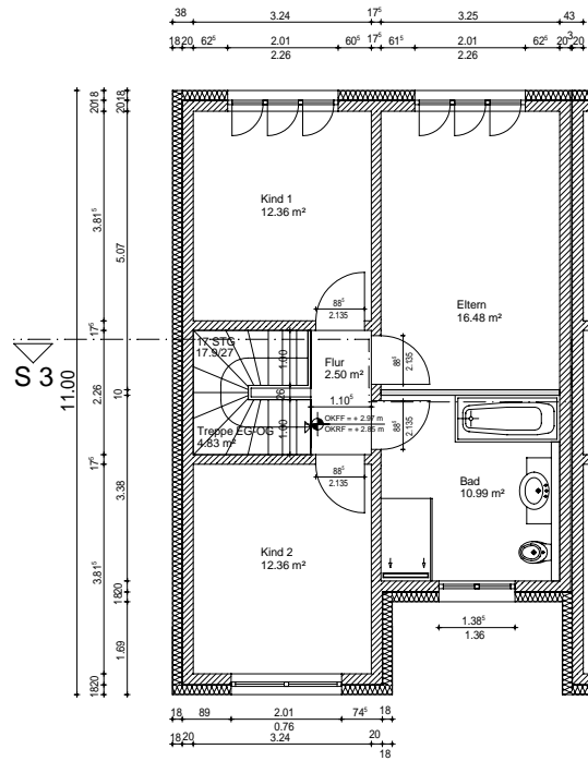
Haus 3 RH 20 - Obergeschoss
